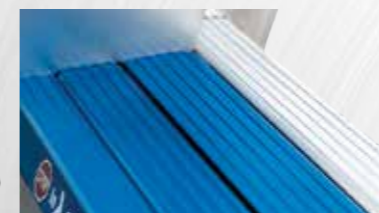
Plattformartige Standflächen im Bereich der Überlappung (115 mm)
